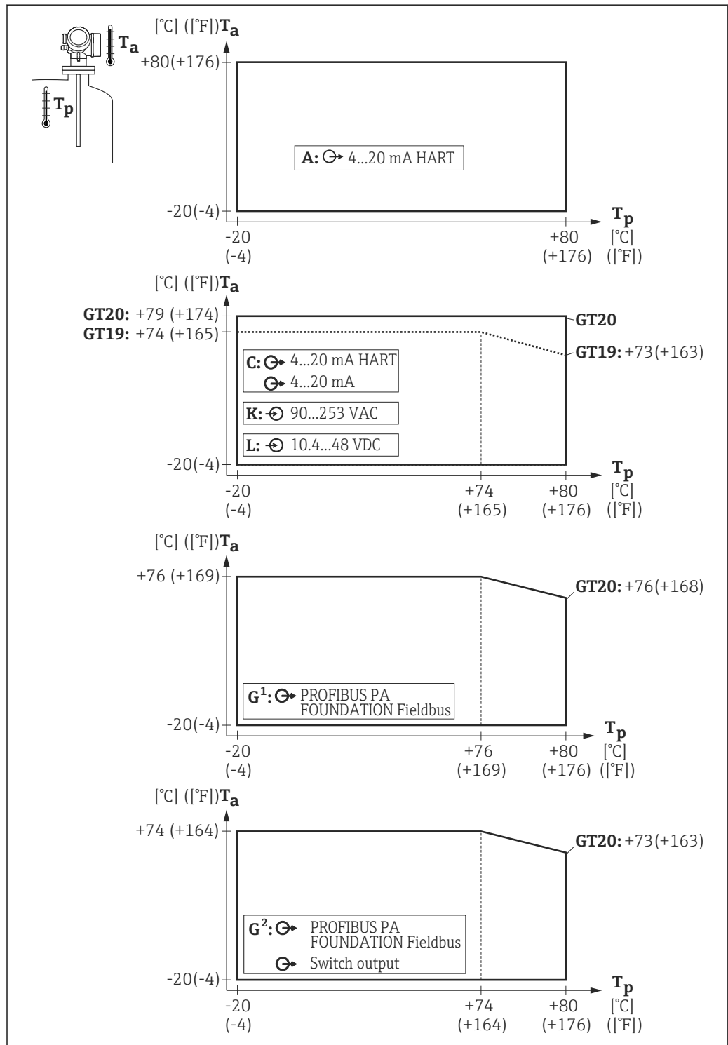
温度曲线: FMP50, 带 G \frac{3}{4} 或 NPT \frac{3}{4} 螺纹连接
