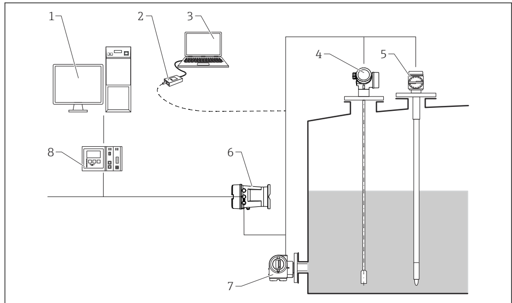
图 40 整套测量系统包括:
