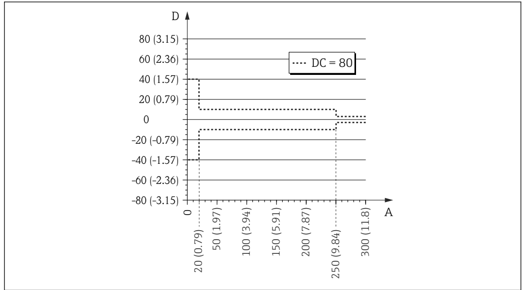
22 缆式探头底部的测量误差
