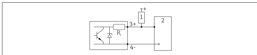
图 18 连接数字量输入
