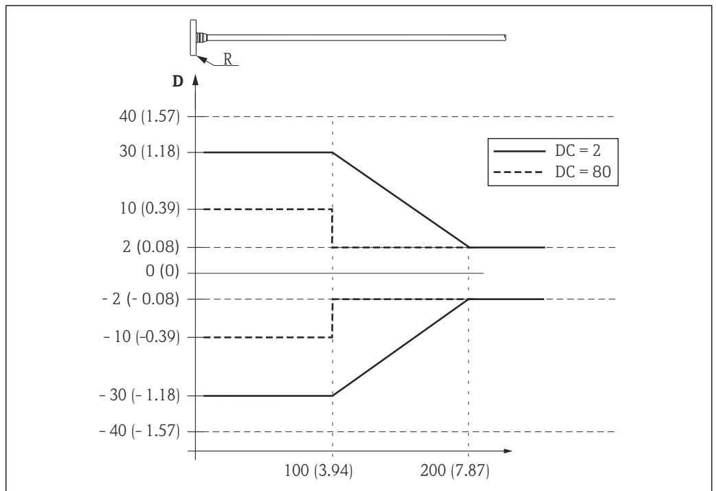
23 探头顶部出现的测量误差; 单位: mm (in)
