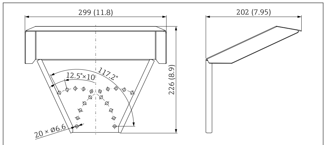
图 44 外形尺寸。测量单位 mm (in)
