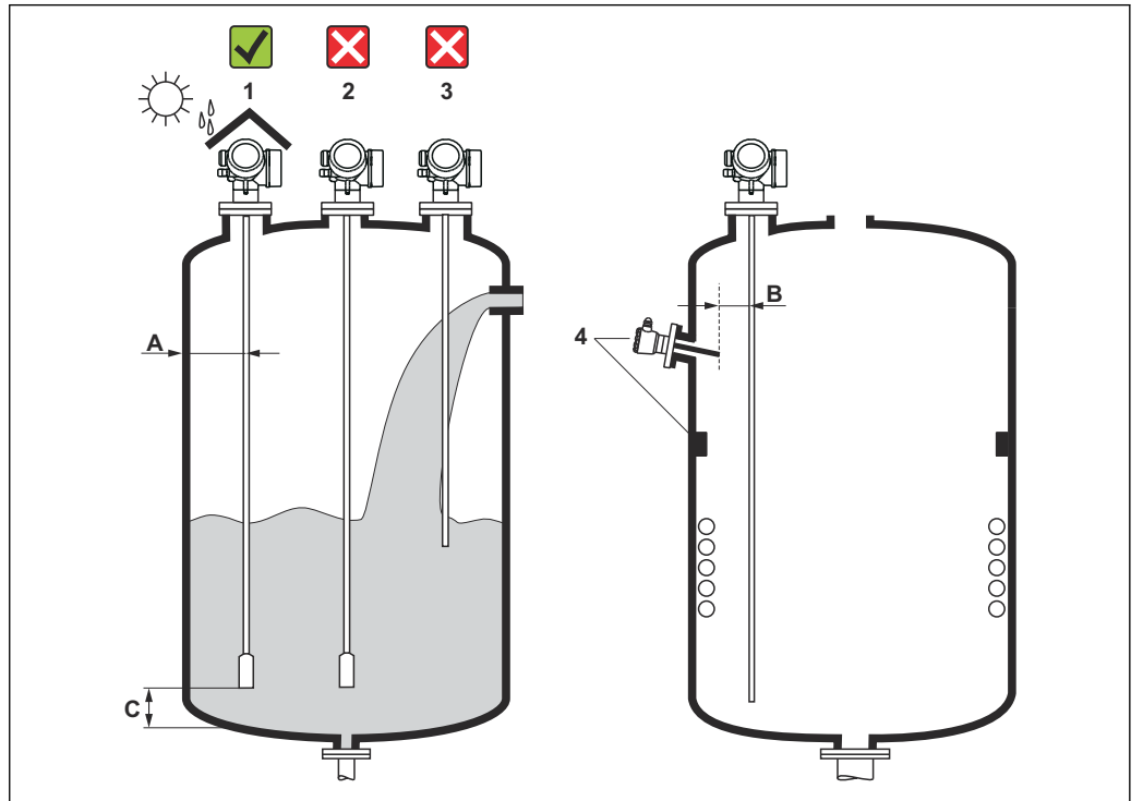
图 24 Levelflex 的安装条件
