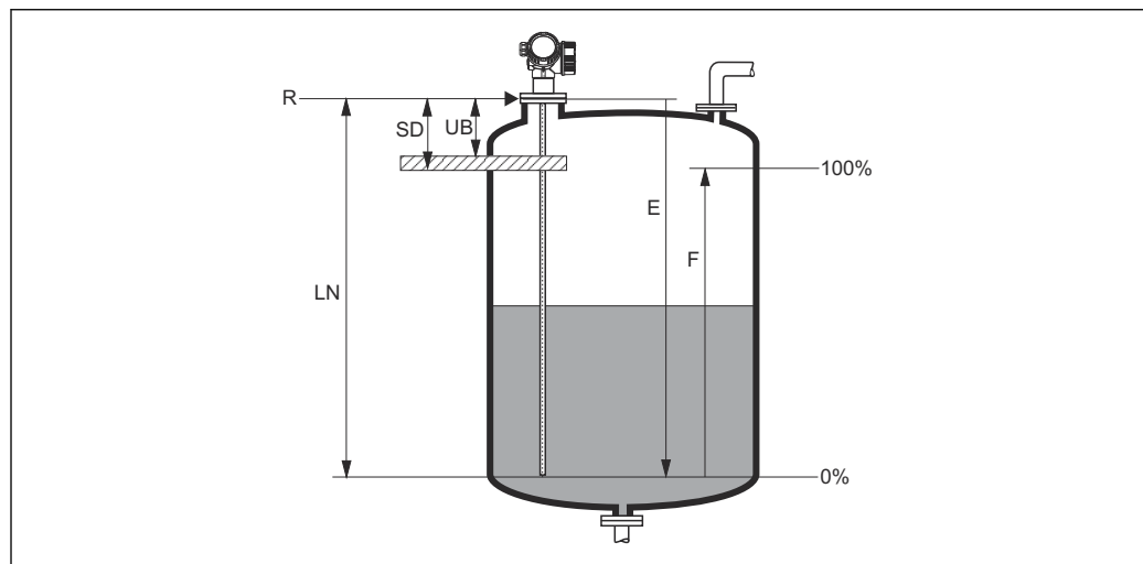
图 4 确定盲区距离和安全距离
