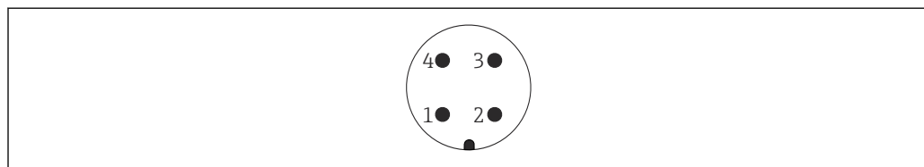
图 19 M12 插头的针脚分配
