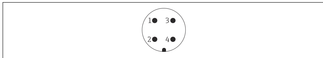
图 20 7/8"插头的针脚分配
