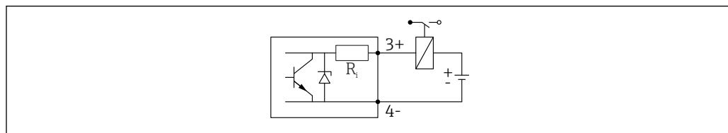
图 17 连接继电器
