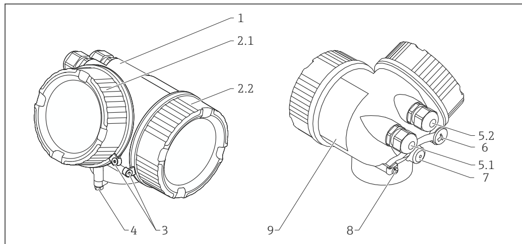
图 33 材质: GT20 外壳
