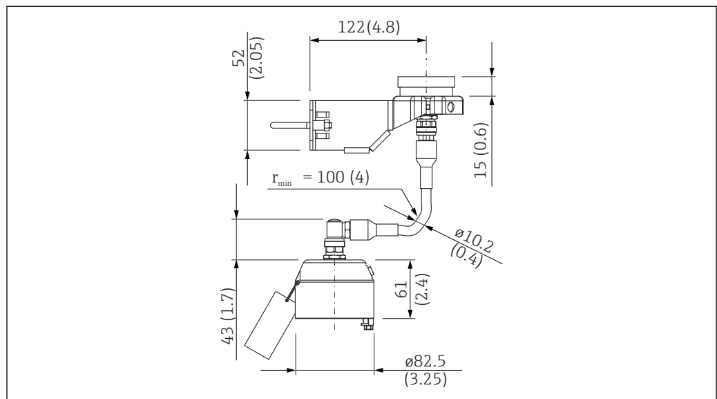
图 30 分体式探头的连接尺寸；连接电缆长度为订购长度。测量单位 mm (in)
