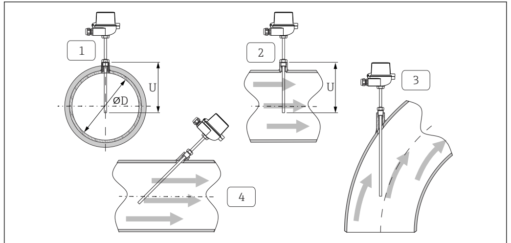
图 7 安装实例
