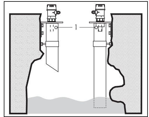
1 通风孔
